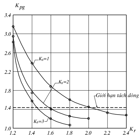
Hình 8-10. Hệ số khí hoá phân giới K_{pg} của các cửa vào elip
