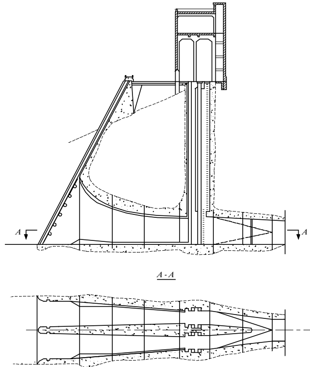
Hình 8-32. Cửa lấy nước kiểu giếng đứng
