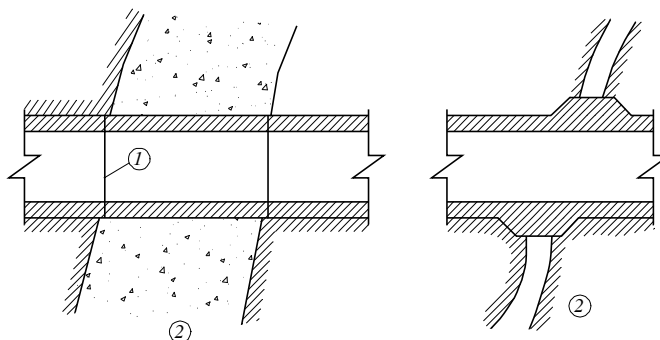
Hình 8-31. Xử lý khi đường hầm xuyên qua các tầng đá đứt gãy
