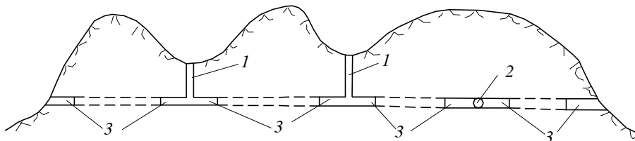
Hình 8-3. Cắt dọc tuyến đường hầm
