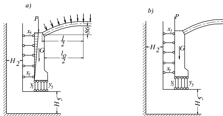
Hình 8-24. Tường bên đàn hồi
