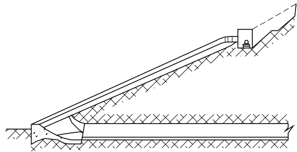
Hình 8-33. Cửa lấy nước kiểu mái nghiêng
