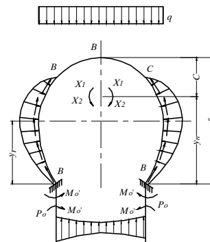
Hình 8-21. Sơ đồ tính toán vòm khép kín
