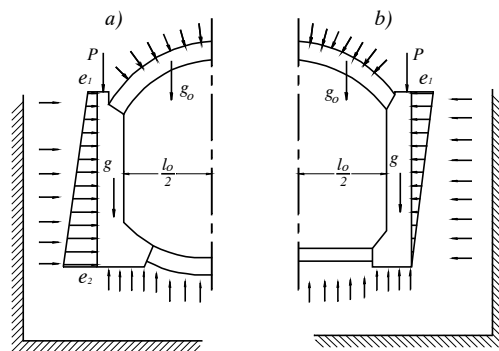
Hình 8-22. Các lực tác dụng lên tường bên
