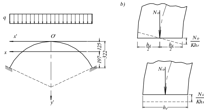
Hình 8-17. Sơ đồ tính toán vòm thấp
