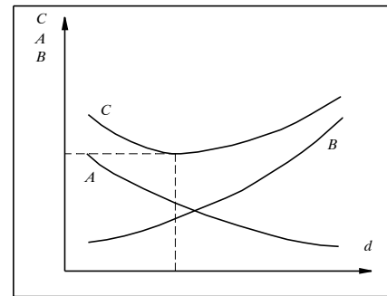
Hình 8-11. Để xác định đường kính kinh tế của đường hầm thủy điện
