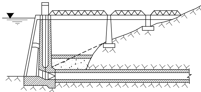
Hình 8-34. Tháp kiểu kín
