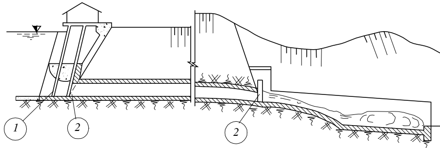
Hình 8-37. Các hình thức bố trí cửa van
