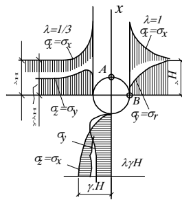
Hình 8-27. Phân bố ứng suất trong khối đá có lỗ khoét tròn khi \lambda = \sigma_x / \sigma_y
