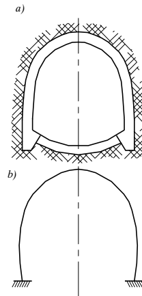
Hình 8-18. Sơ đồ tính toán vòm cao
