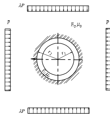
Hình 8-28. Sơ đồ tác dụng của tải trọng lên khối đá bao quanh lớp lót đường hầm
