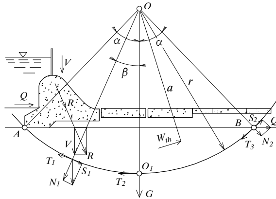
Hình 2-27. Sơ đồ tính toán ổn định đối với mặt trượt trụ tròn giới hạn, nền đồng nhất
