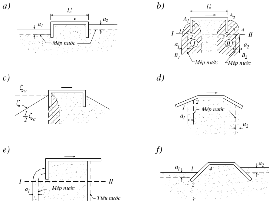
Hình 2-16. Đơn giản hóa các dạng hình học của trụ biên
