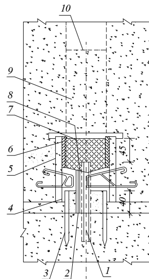
Hình 2-7. Liên kết bản cừ với bản đáy sử dụng đến chốt
