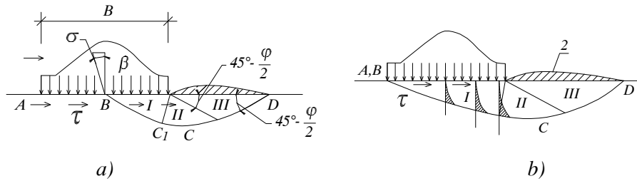
Hình 2-26. Sơ đồ sự dịch chuyển cung trượt sâu và trượt hỗn hợp
