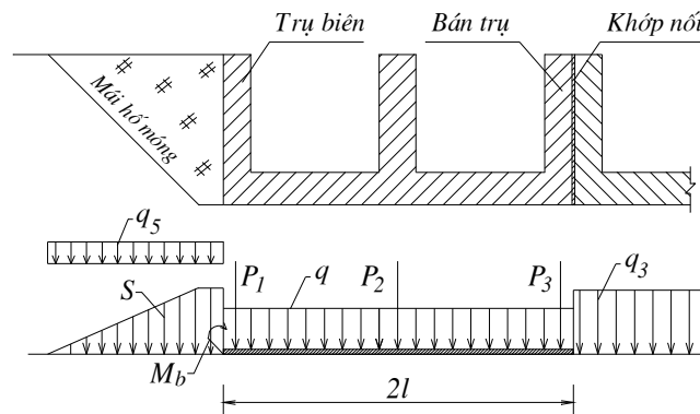
Hình 2-34. Sơ đồ ngoại lực cuối cùng tác dụng lên dải bản đáy
