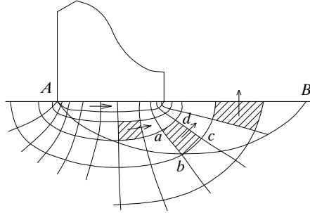
Hình 2-28. Sơ đồ tính toán lực thấm W_{th}
