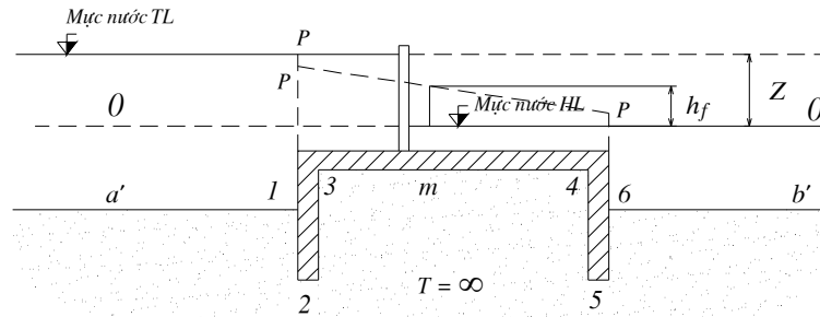
Hình 2-17. Tắm đáy tương đương (có độ bền thấm tương đương với trụ biên đang xét)
