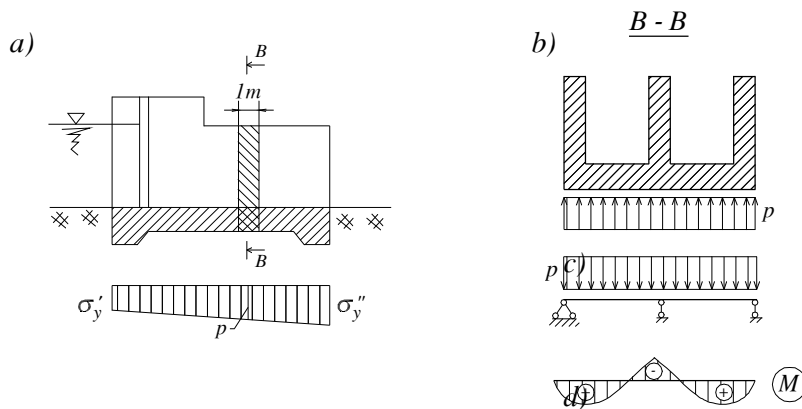
Hình 2-32. Sơ đồ tính toán bản đáy đập theo phương pháp dầm đảo ngược
