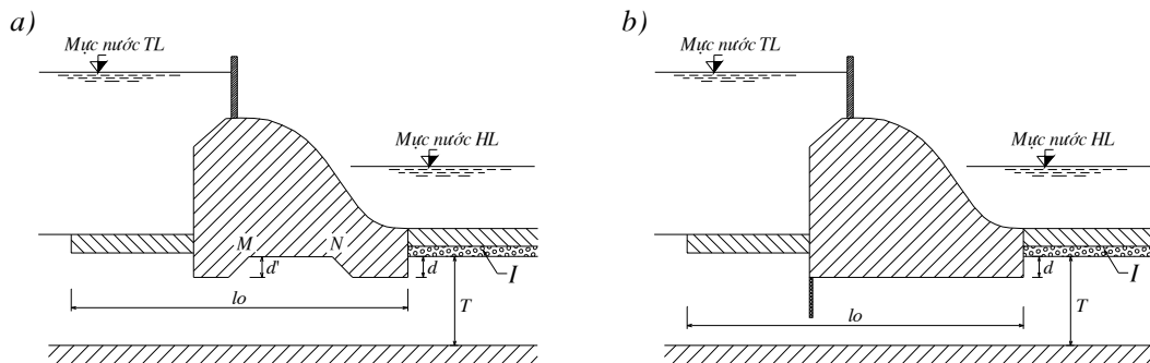
Hình 2-9. Thiết kế móng đập
