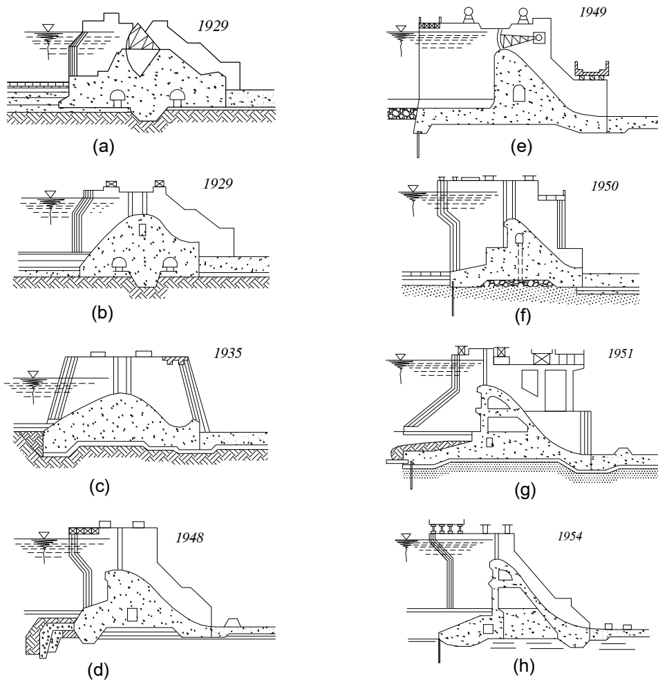
Hình 2-2. Một số đập tràn trên nền mềm được xây dựng ở Liên Xô (cũ) từ năm 1929 đến 1954
