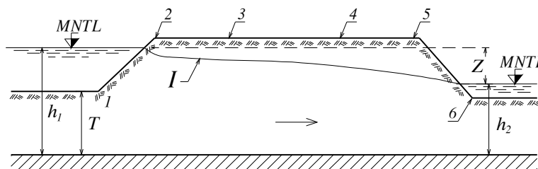
Hình 2-12. Đường bão hòa quanh trụ biên-I
