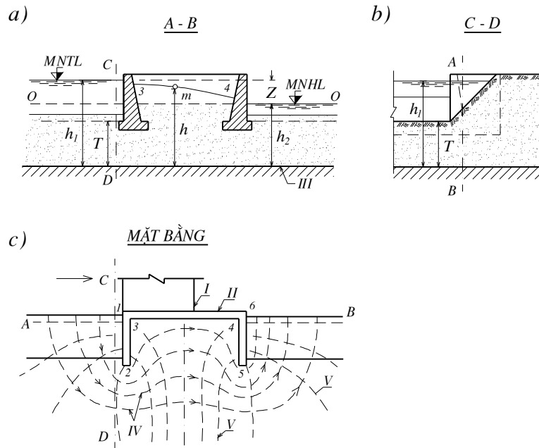
Hình 2-11. Trụ biên có tường cánh thẳng góc
