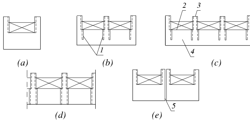
Hình 2- 20. Phân chia đập thành các đơn nguyên
