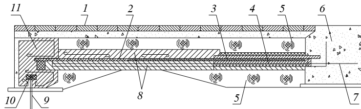
Hình 2-6. Sơ đồ sân trước neo
