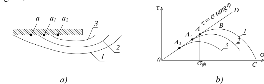
Hình 2-25. Sơ đồ tính toán trượt sâu và trượt hỗn hợp
