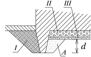
Hình 2-8. Chân khay thượng lưu dưới đập
