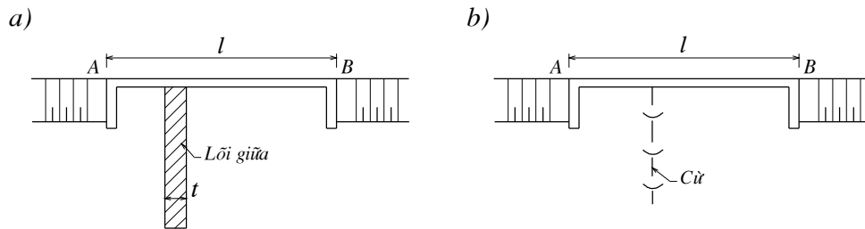
Hình 2-18. Trường hợp trụ biên nối tiếp với lõi giữa bằng đất sét hoặc màng ngăn dưới dạng hàng cừ
