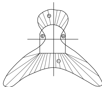
Hình 1-25. Ứng suất tập trung quanh đường hãm
