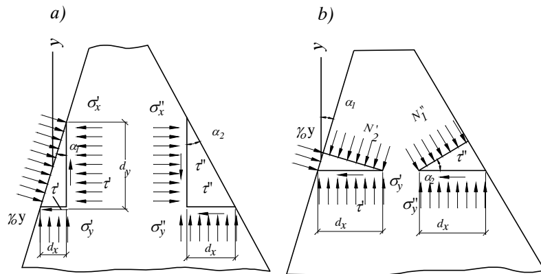
Hình 1-11. Sơ đồ xác định các loại ứng suất ở biên đập
