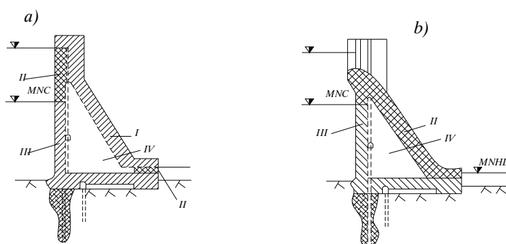
Hình 1-36. Phân vùng vật liệu thân đập
