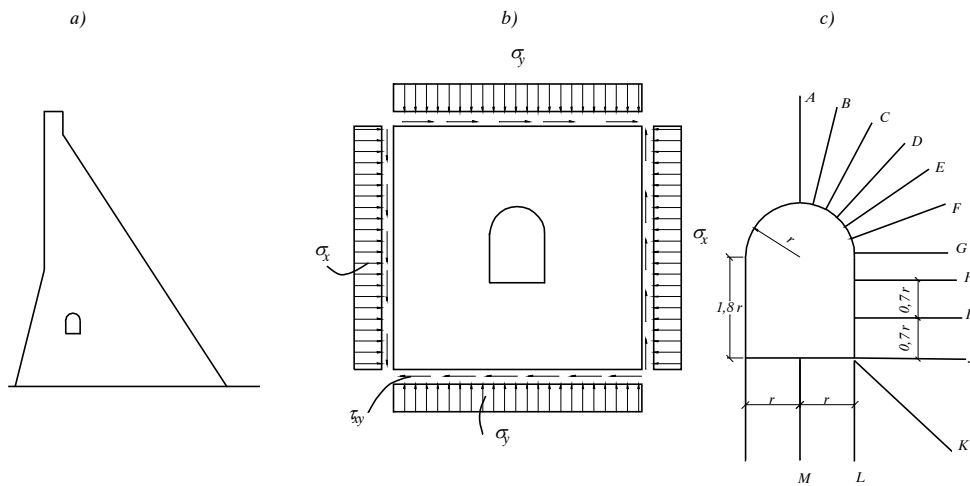
Hình 1-24. Sơ đồ tính toán ứng suất quanh đường hãm tiêu chuẩn
