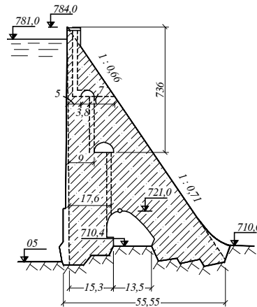
Hình 1-38. Đập có lỗ lớn ở nền
