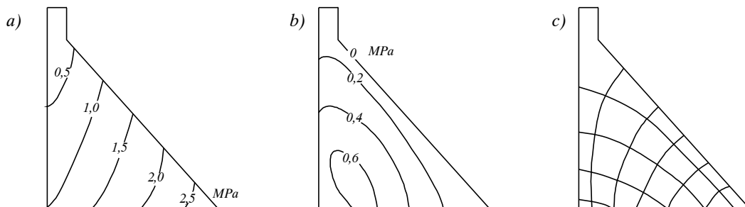
Hình 1-14. Các đường đẳng ứng suất, quỹ đạo ứng suất
