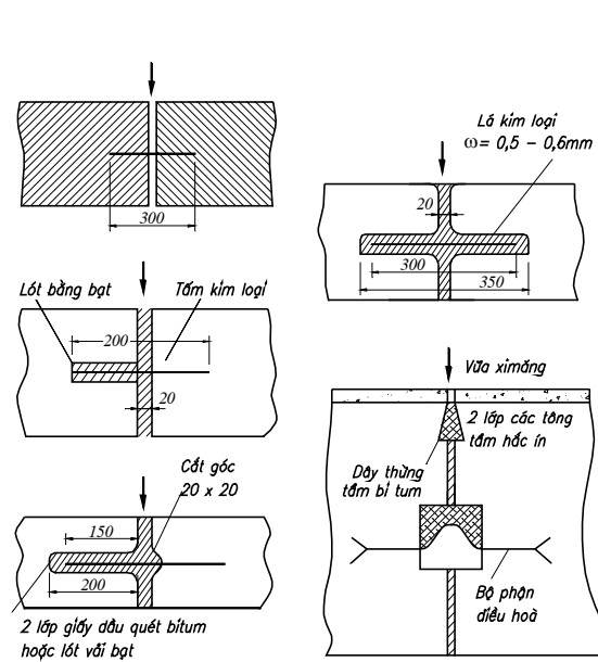
Hình 1-34. Các kiểu khớp nối chống thấm bằng các tấm kim loại
