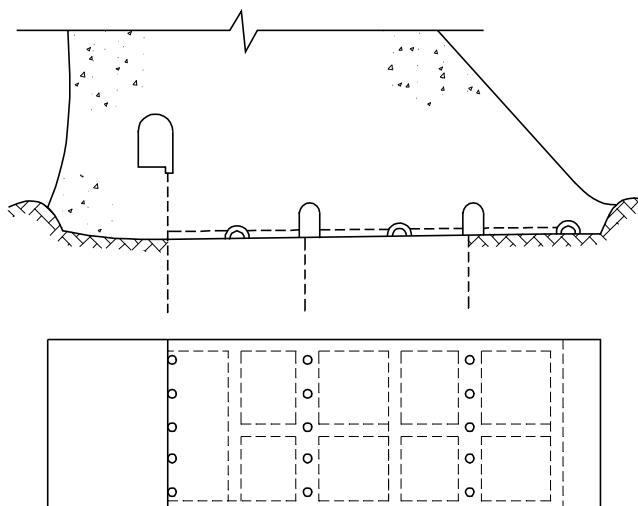
Hình 1-31. Hệ thống thoát nước dưới nền đập
