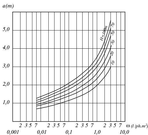
Hình 1-28. Đồ thị xác định khoảng cách giữa các lỗ khoan trong trường hợp đá nền có khe nứt lớn
