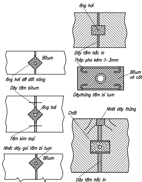
Hình 1-33. Các kiểu khớp nối chống thấm bằng bitum
