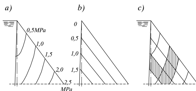
Hình 1-19. Các đường đẳng ứng suất pháp chính
