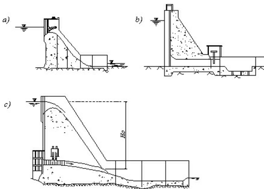
Hình 1-2. Các hình thức đập trọng lực tràn nước
