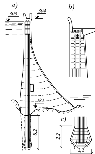
Hình 1-39. Đập có neo ứng suất trước
