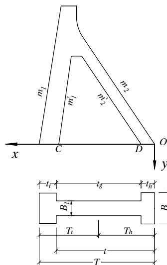
Hình 1-40. Mặt cắt tính toán ứng suất đập khe rộng
