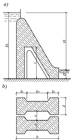
Hình 1-37. Đập trọng lực khe rộng
