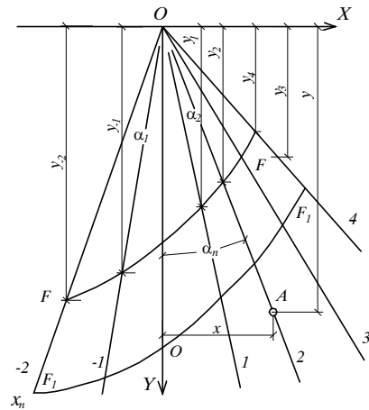
Hình 1-18. Sơ đồ vẽ đường đẳng ứng suất
