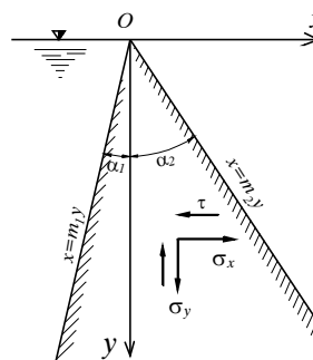
Hình 1-15. Sơ đồ tính ứng suất theo lý thuyết đàn hồi
