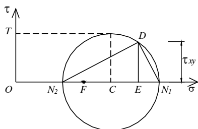
Hình 1-13. Sơ đồ vòng Mo ứng suất tại 1 điểm
