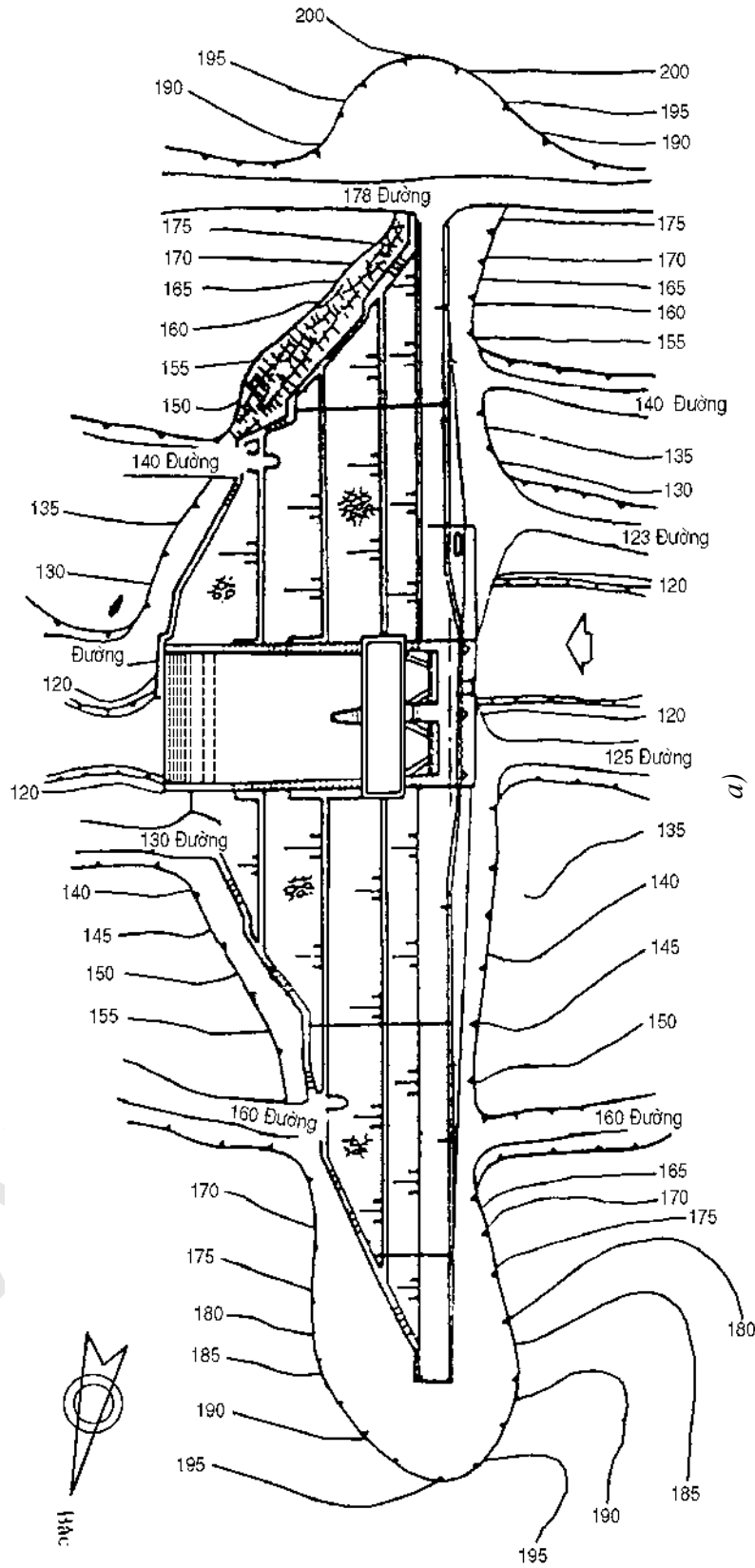
Hình 2-28. Đập trọng lực đá xây Hoàng Long Đồi
