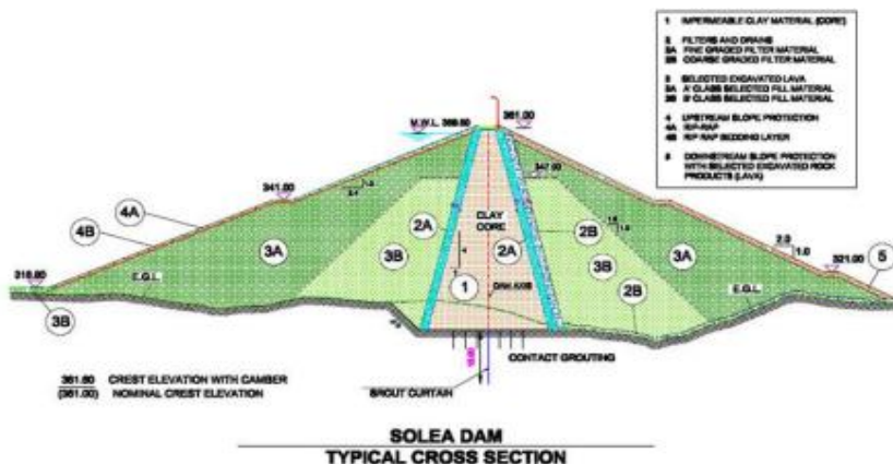
Mặt cắt điển hình của đập Solea (Cyprus)
