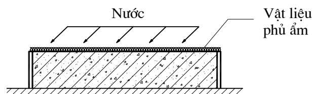
Hình 1- Sơ đồ phủ ẩm bảo dưỡng bê tông
