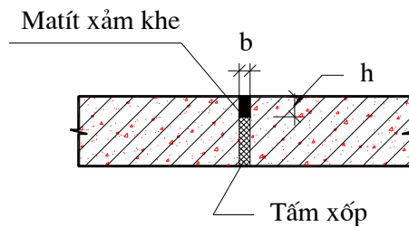
Hình 8- Cấu tạo khe dãn sau thi công.
