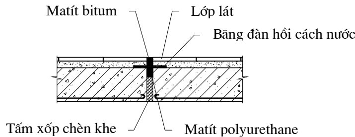
Hình 5- Sơ đồ khe dẫn có nhu cầu ngăn nước cao
