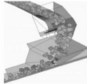
Hình 13. Mô phỏng 3D quá trình vận chuyển đá rời bằng băng tải [13]
