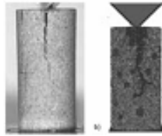
Hình 9. Mô phỏng thí nghiệm nén đập mẫu đá có xét kiến trúc hạt. Nguồn: TUBAF
