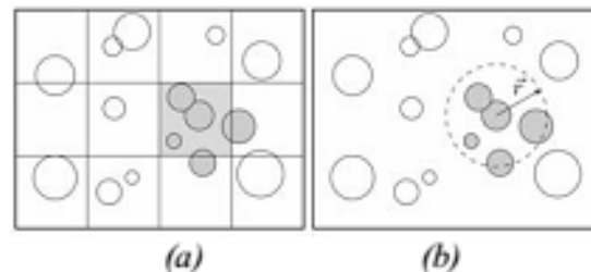
Hình 1. Hệ thống ô lưới quản lý vị trí các phần tử; (b) dò tìm điểm tiếp xúc theo phương pháp Verlet. [2]
